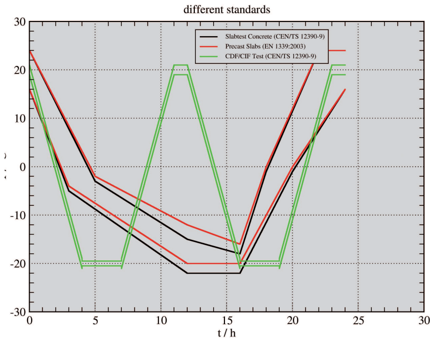
Fig. 2 Curvas de temperaturas referencias según las diferentes normas (Indicadas en el cajetín remarcado).
