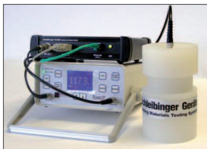
Fig. 9. Equipo de Ultrasonidos para medida de las retracciones. A la dcha. Sensor de US para morteros, a su lado el aparato de medida y registro de la retracción; y encima el Datalogger (interface).
