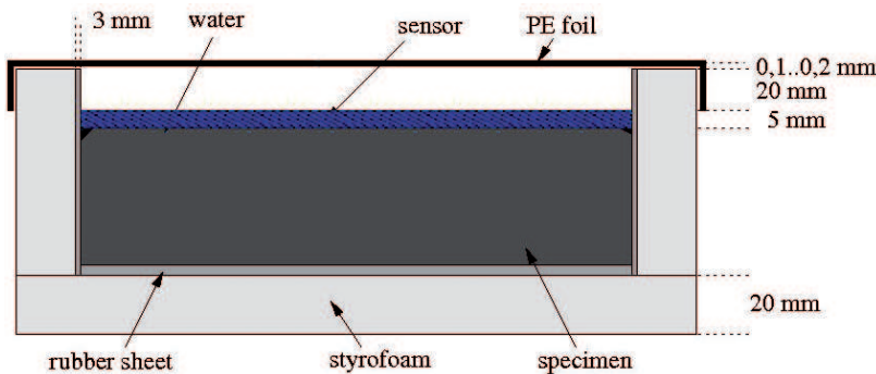
Fig. 3 Aislamiento del cubo para garantizar helada uniaxial.
