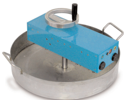
Fig. 11. Reómetro BT 2 de hormigón fresco.
